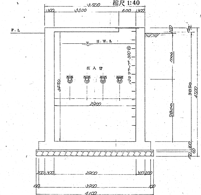
C-C 断面図 縮尺 1:40
