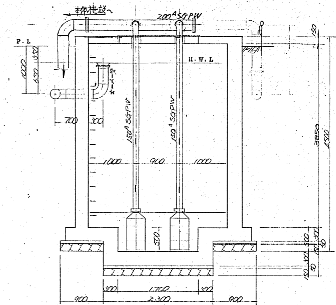
C-C 断面図 縮尺 1:40
