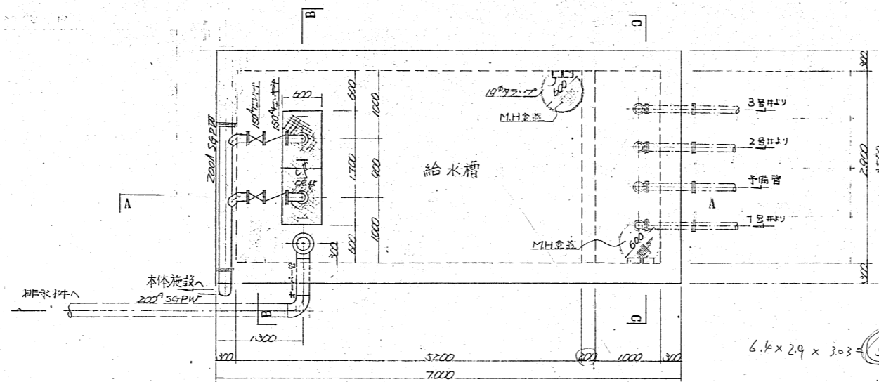
平面図 縮尺 1:40
