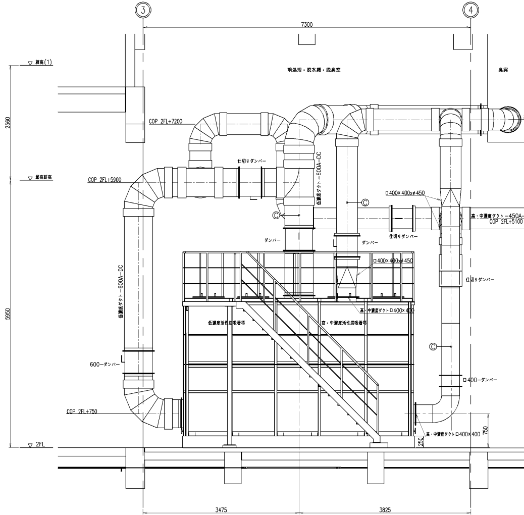
D-D 矢視
