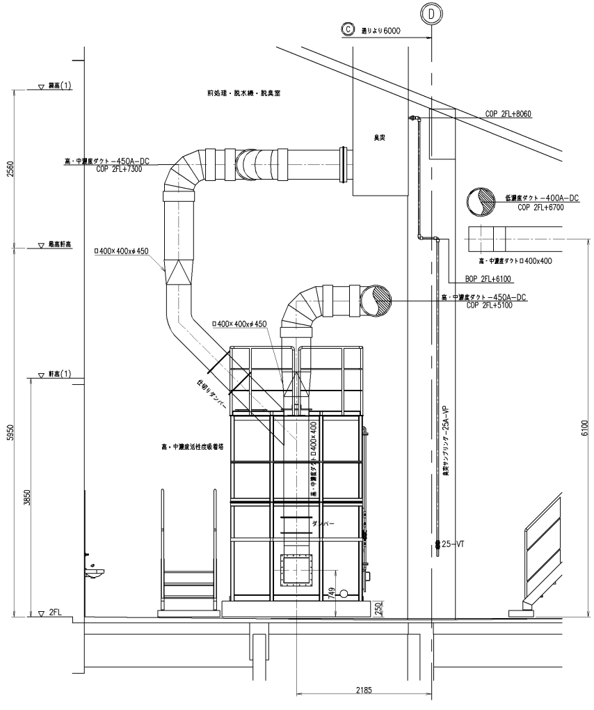
E-E 矢視
